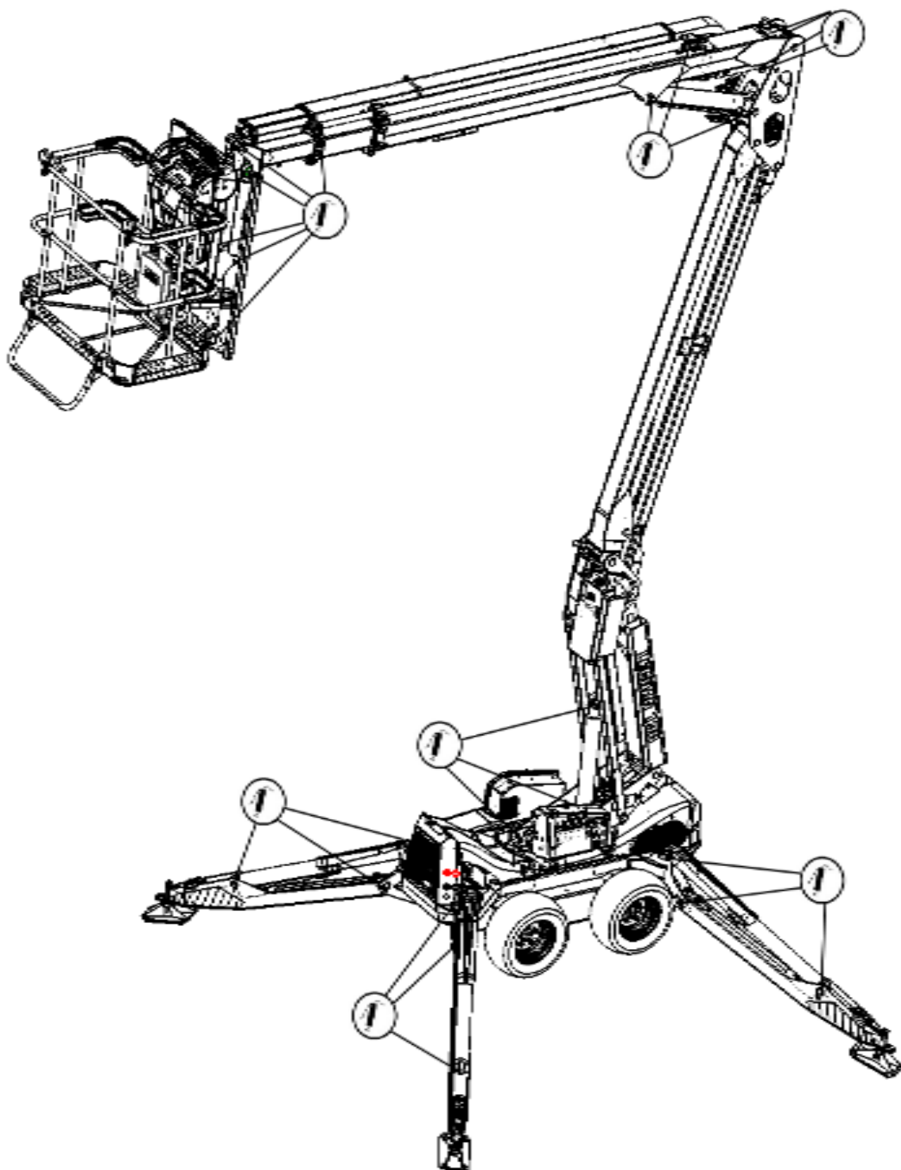
Figura 18: Esquema de engrase
