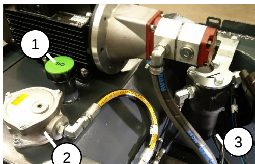
Figura 20: Filtros de aceite hidráulico
