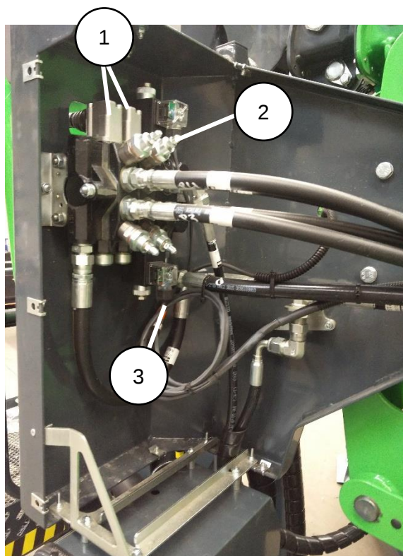
Figura 25: Carcasa de la válvula de pedestal
