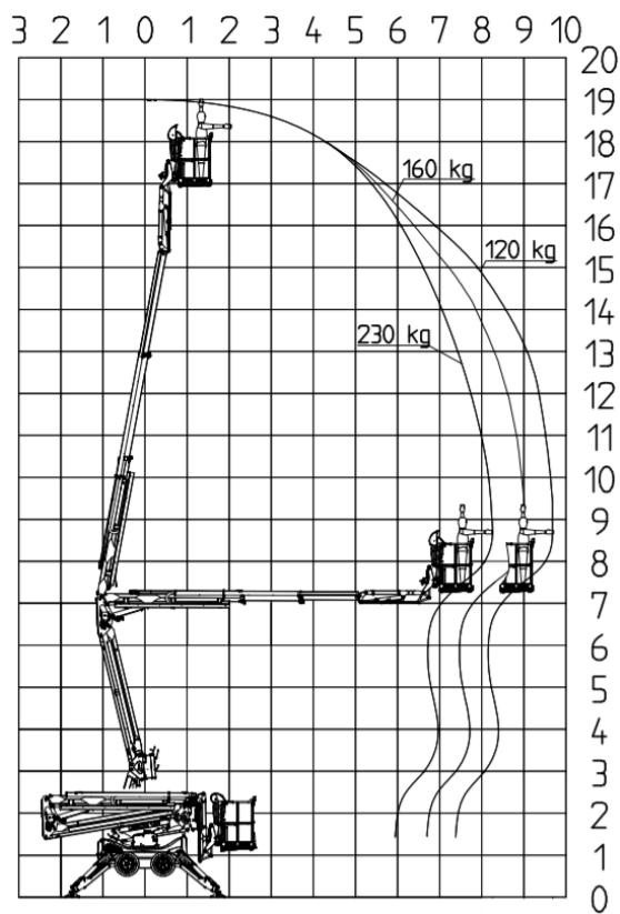
Figura 2: Diagrama de alcance
