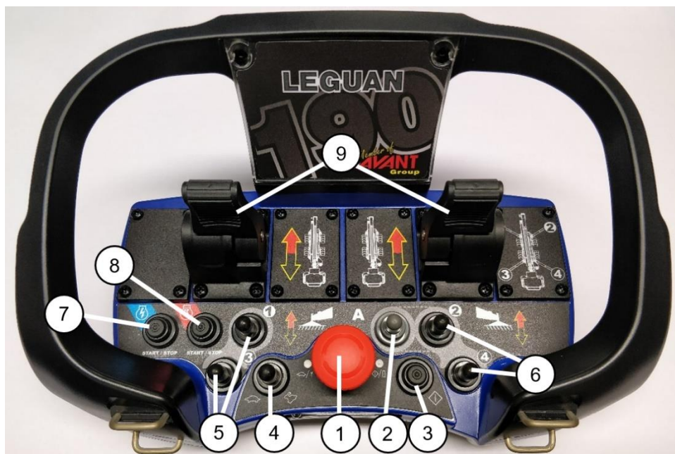
Figura 8: Control remoto inalámbrico
