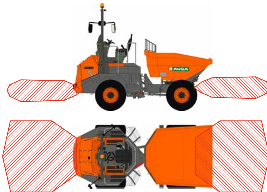
Alcance del FVS
