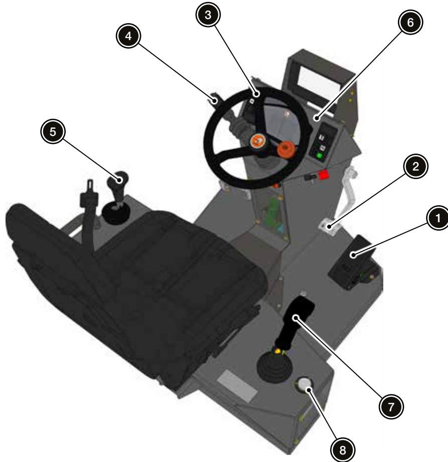
Panel de mandos
