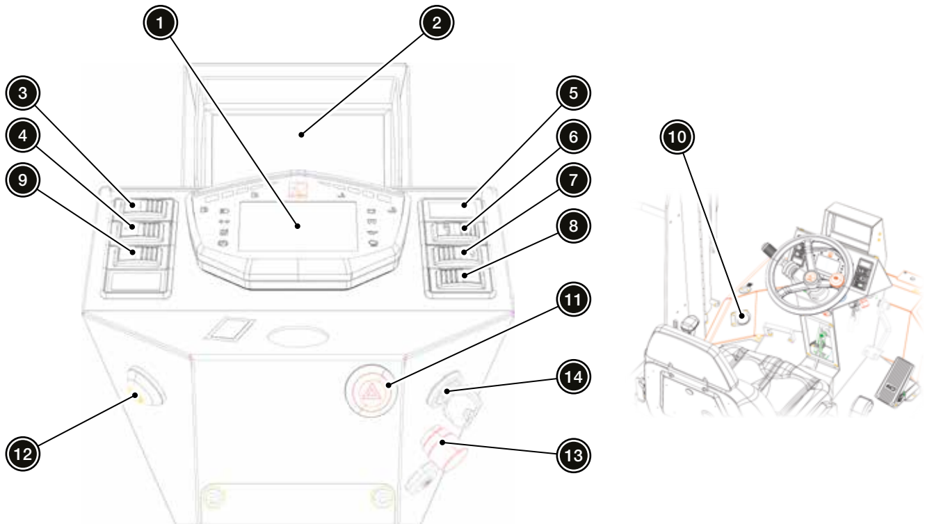
Cuadro de instrumentos
