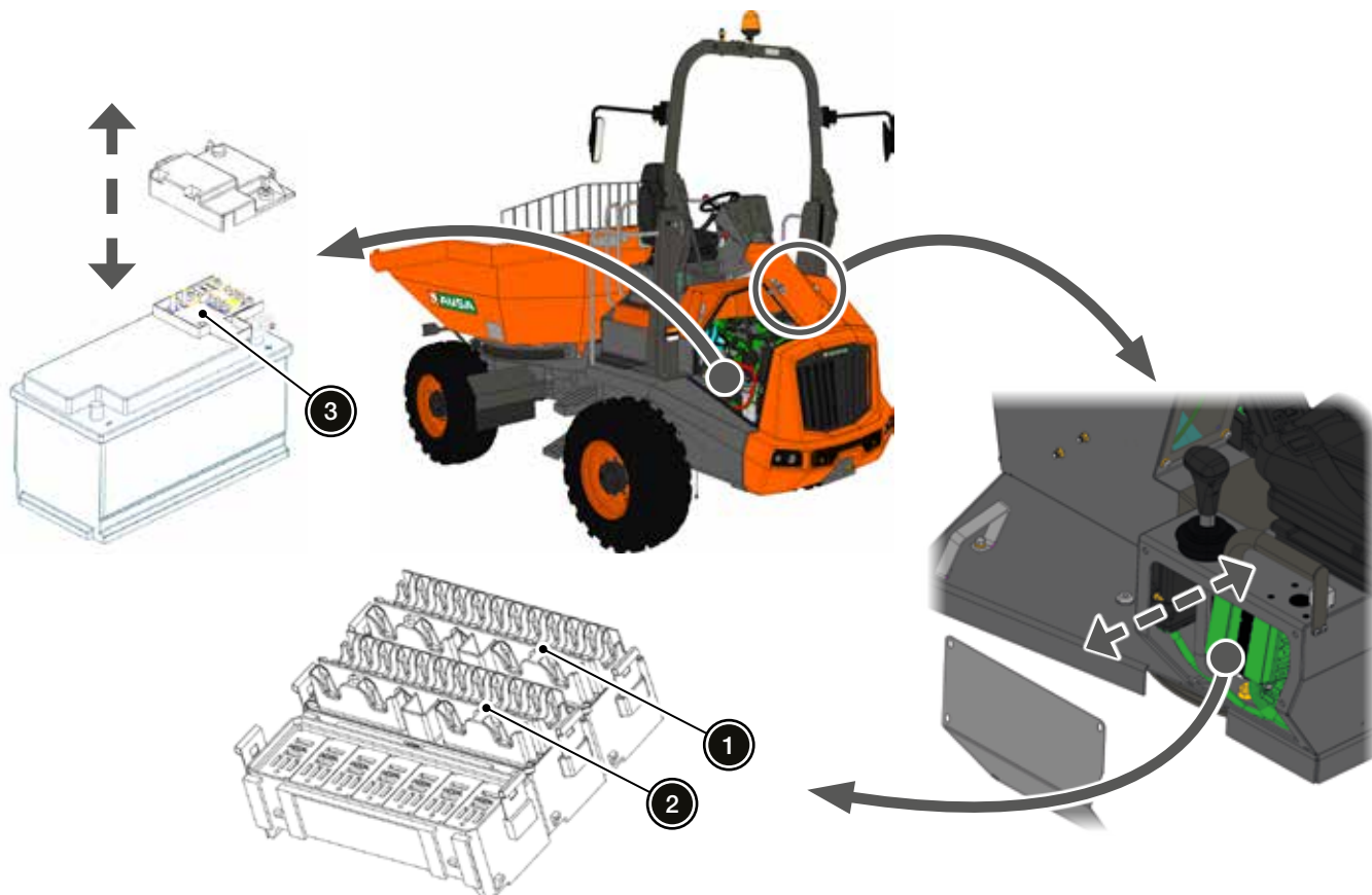
Ubicación de las cajas de fusibles
