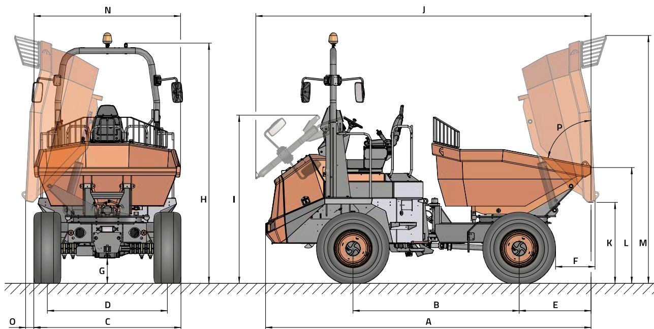
Dimensiones y alcance de la máquina
