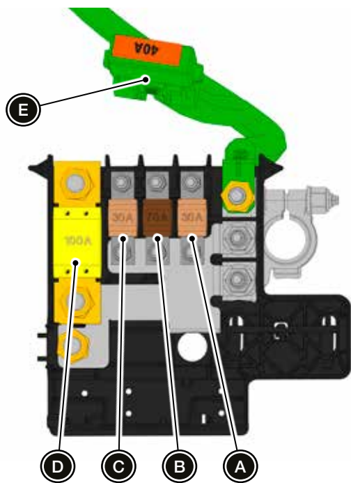
Caja de fusibles 3
