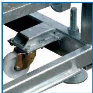
Detalle de la base Base-frame detail
