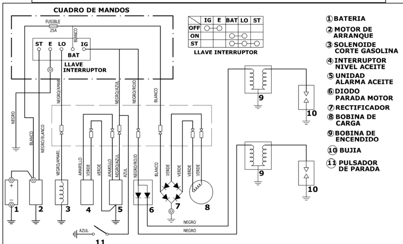
ESQUEMA ELECTRICO COBRA-60-G20H
